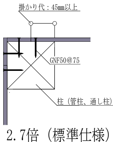
図7 出隅部（外面合わせ）の納まり図
