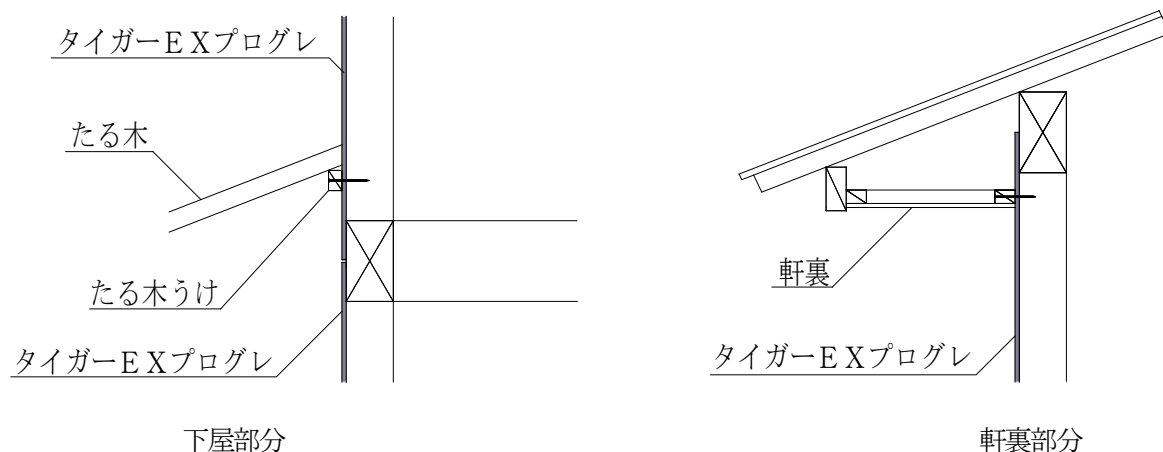
図9 下屋、軒裏納まり図
