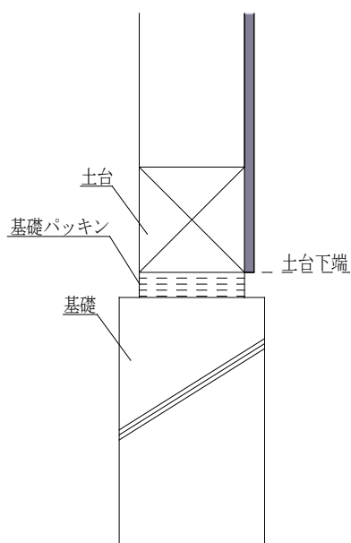
図8 土台部の納まり図
