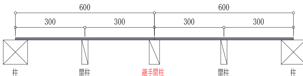
図14 2Pの壁 納まり図
