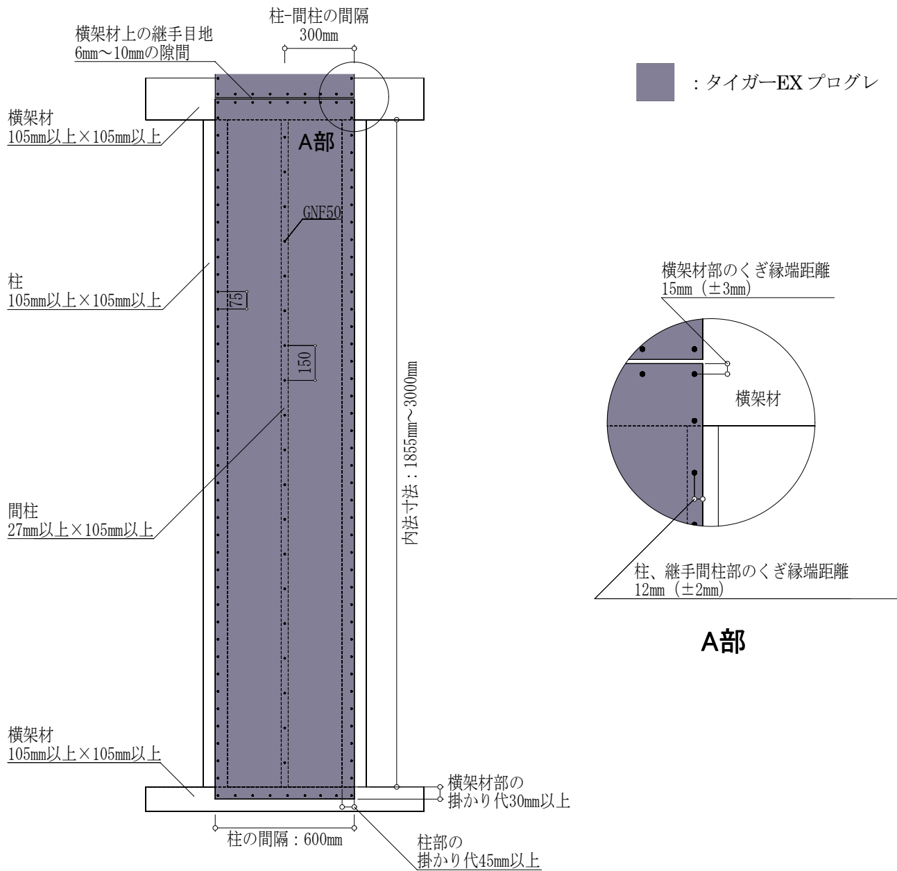
図6 標準仕様（FRM-0780：2.7倍） 施工概略図
