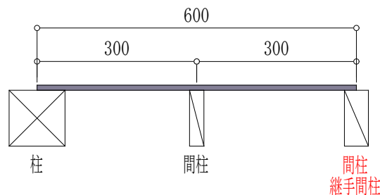
図 15 端部が間柱および継手間柱の壁 納まり図
