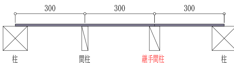
図13 1.5Pの壁 納まり図
